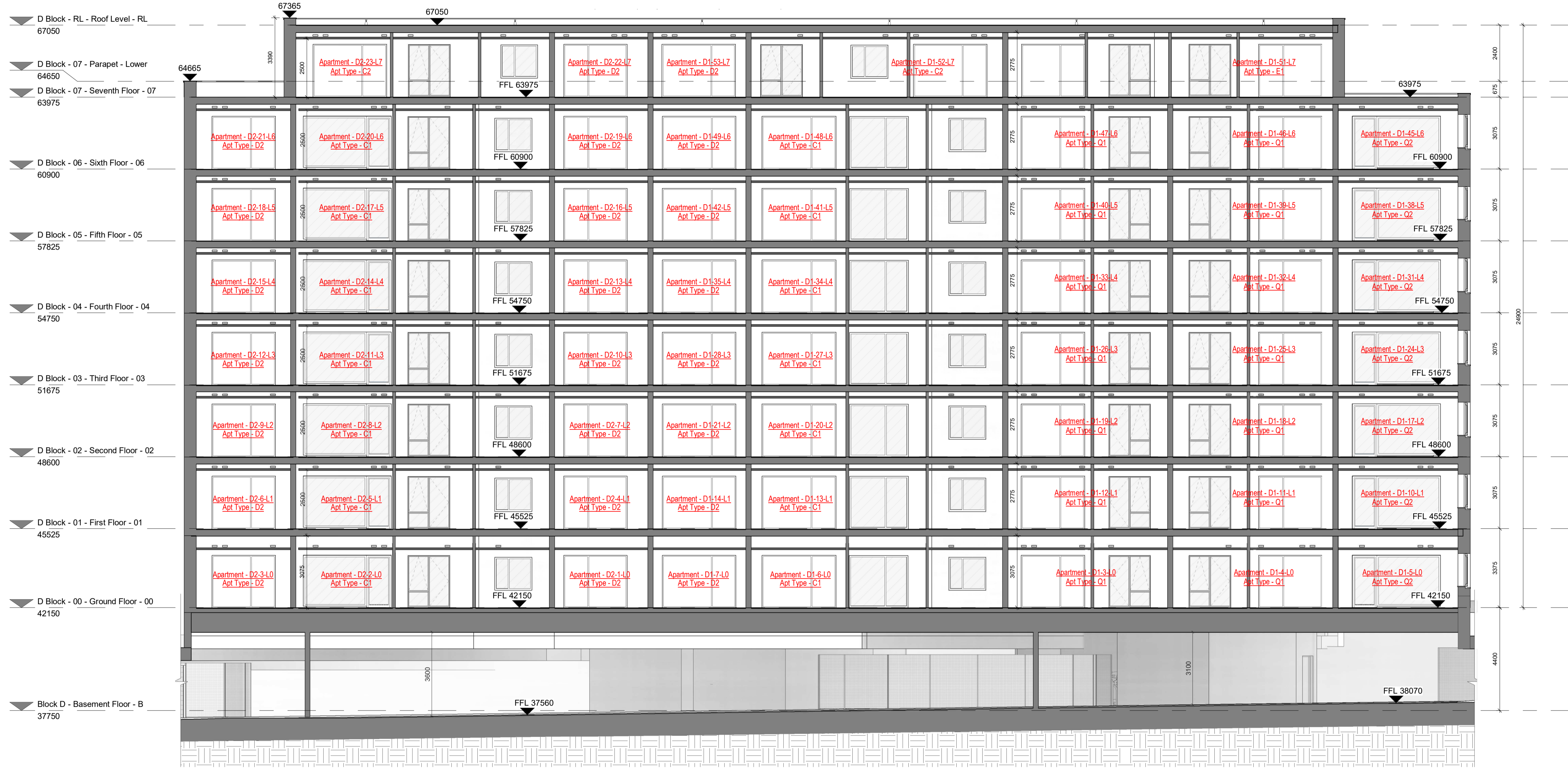
1 GA - Section DD 1 : 100
